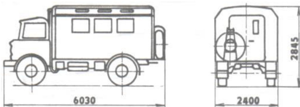
Rozměrové schéma GAZ– 66 K
